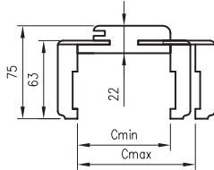
Prierez OR, ORC zo zásuvnou časťou K63
